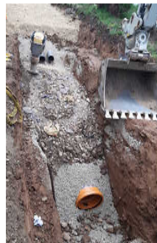
Der Abwasserkanal (orangefarbenes Rohr) wurde aufdimensioniert und zusätzlich wurden Leerrohre (schwarze Rohre) eingelegt.
